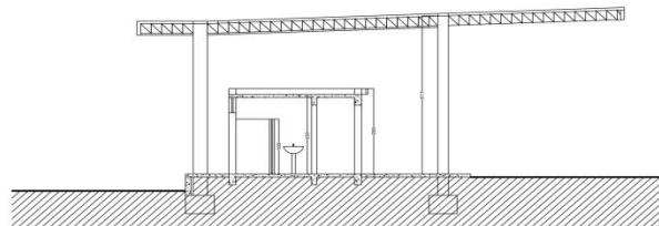
Corte B-B escala 1:75
