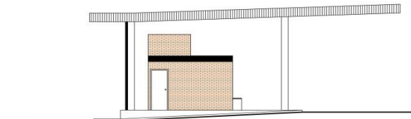
FACHADA LATERAL ESQUERDA escala 1:75
