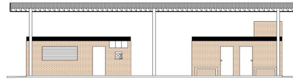
FACHADA FRONTAL escala 1:75
