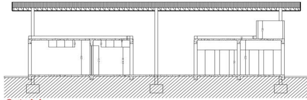
Corte A-A escala 1:75
